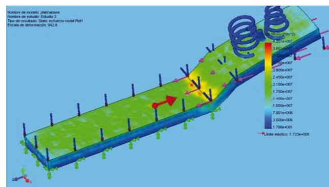
Figura 6. Análisis de esfuerzos base-resorte
