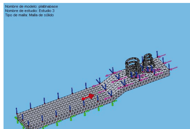
Figura 5. Modelo de base enmallado en sólidos tetraédricos.
